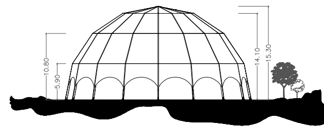
HAUPTANSICHT
