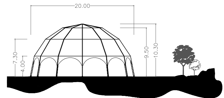
HAUPTANSICHT
