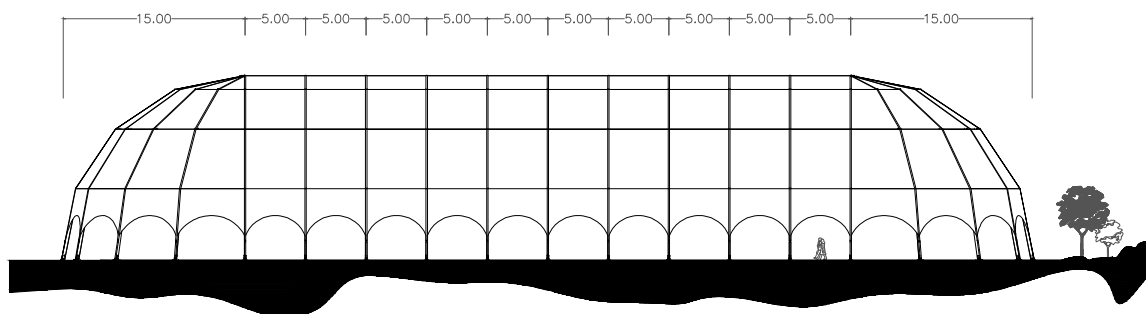
SEITENANSICHT
