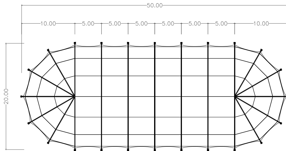
DRAUFSICHT
