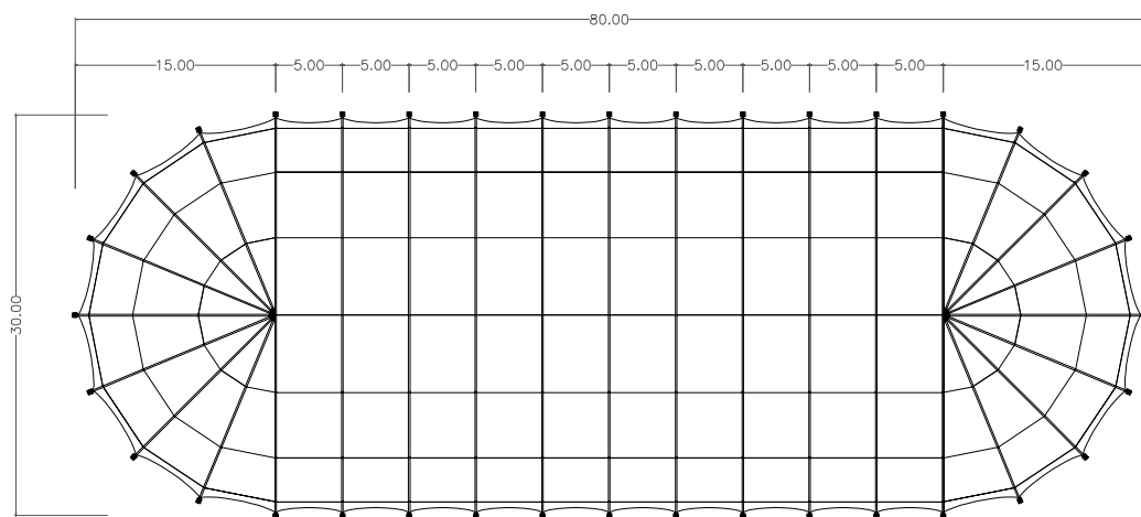
DRAUFSICHT
